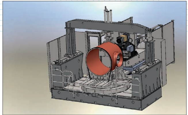
Модель монтажной платформы в T-FLEX CAD
